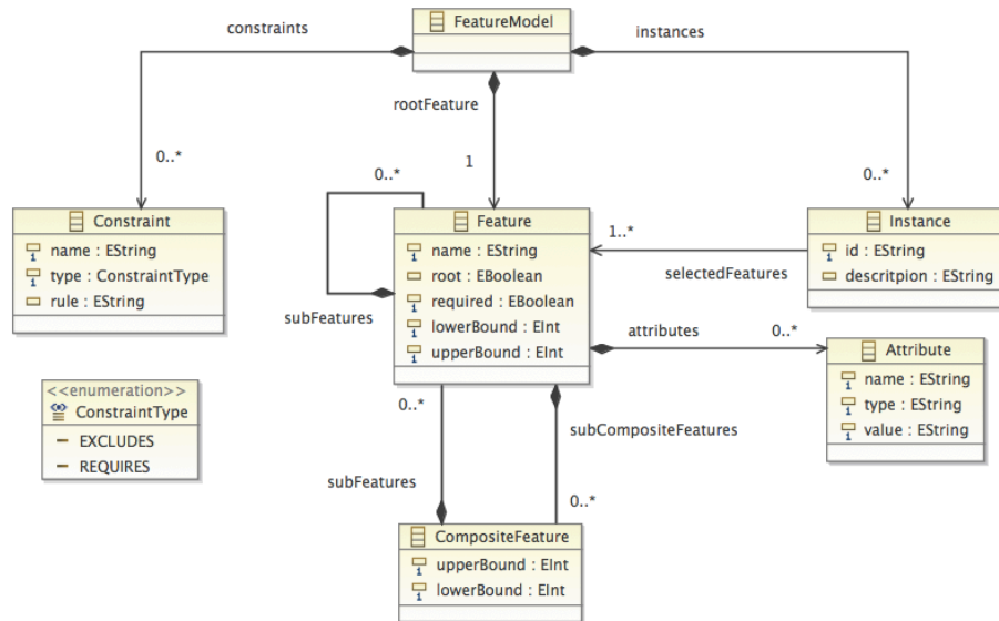
Fig. 2. The Meta-Model
